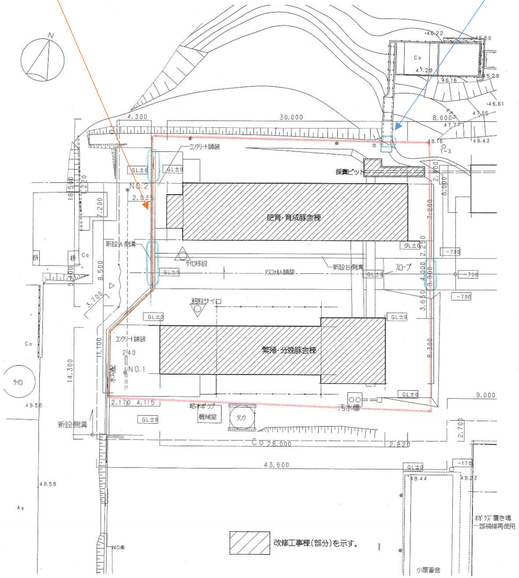
豚舎改修配置図 S=1/300
